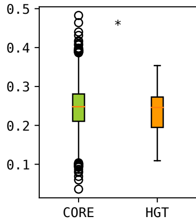
CBI
