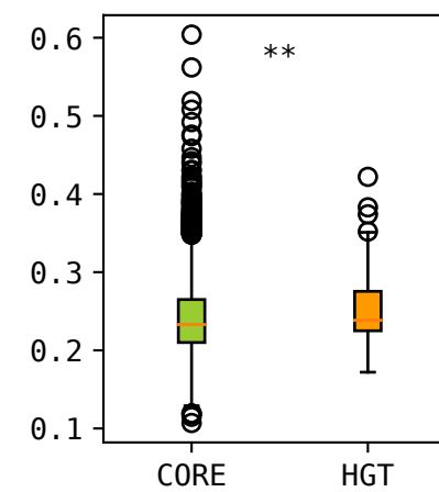
GC
